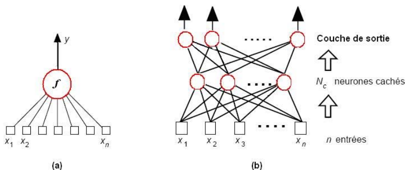
Figure 1 : Le neurone formel et le réseau multicouche
