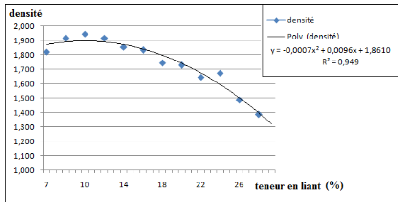
Figure 6 : Variation de la densité en fonction de la teneur en liant
